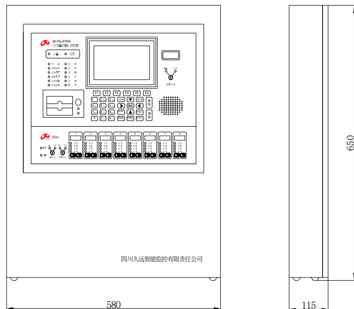
JB-TB-JF999-H 火灾报警联动控制器消防联动控制器外形图
